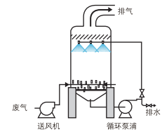
废气洗涤塔
